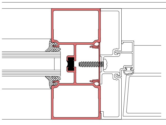
JAMB DETAIL
